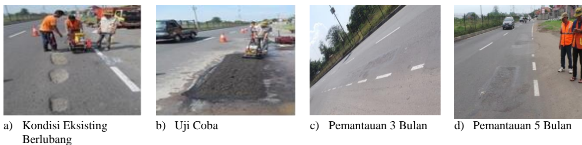
Gambar 17 Hasil uji coba di Ruas jalan Cirebon-Cikampek arah Cikampek KM 19+500
