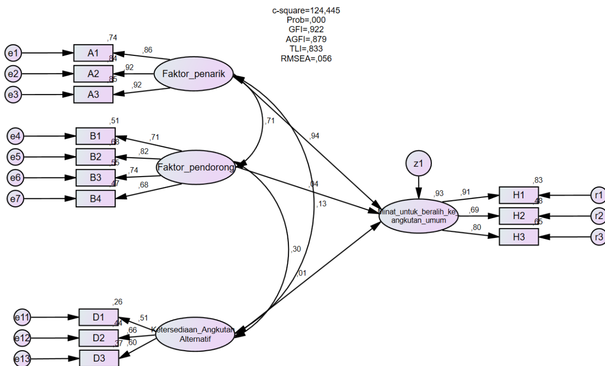
Gambar 5. Model Struktural Terbaik
