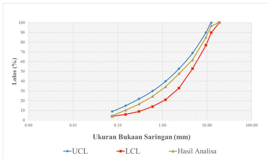
Gambar 1 Gradasi Gabungan
