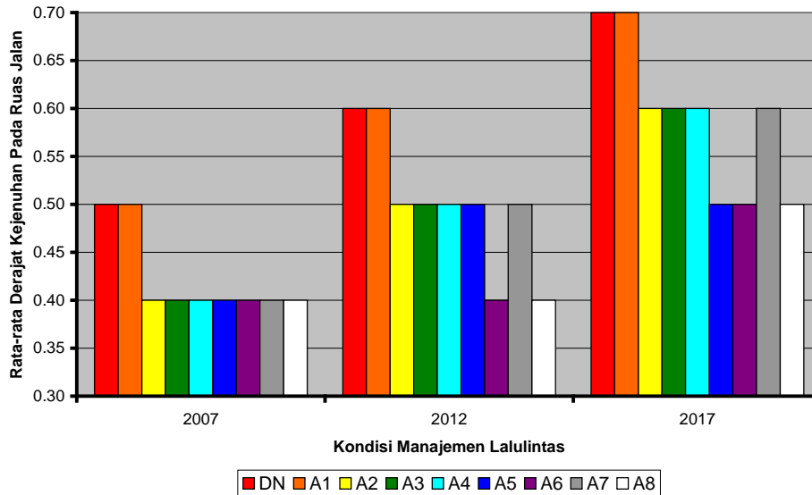
Gambar 11 Perbandingan Derajat Kejenuhan Rata-Rata Pada Ruas Jalan untuk Tahun 2007 Hingga Tahun 2017
