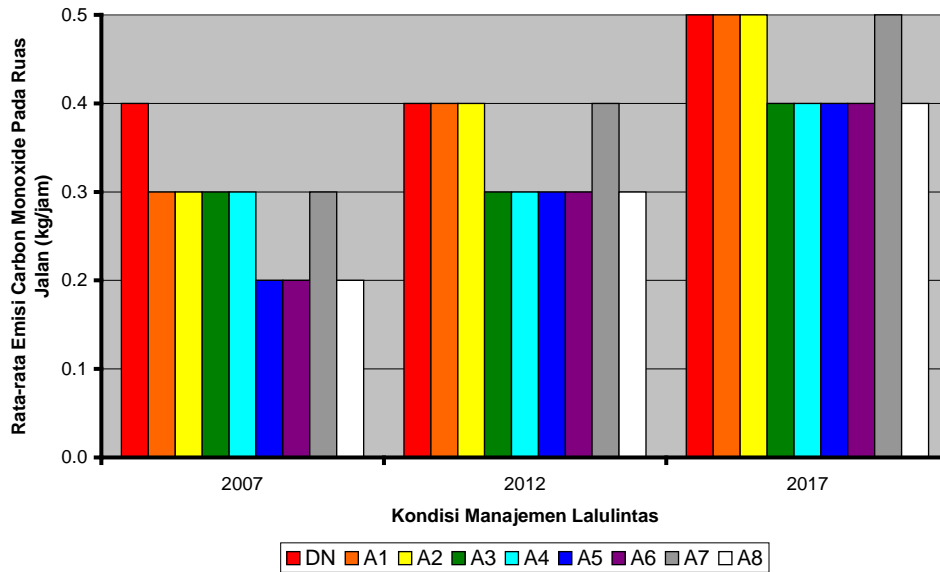
Gambar 13 Perbandingan Emisi Carbon Monoxide Rata-Rata Pada Ruas Jalan untuk Tahun 2007 Hingga Tahun 2017
