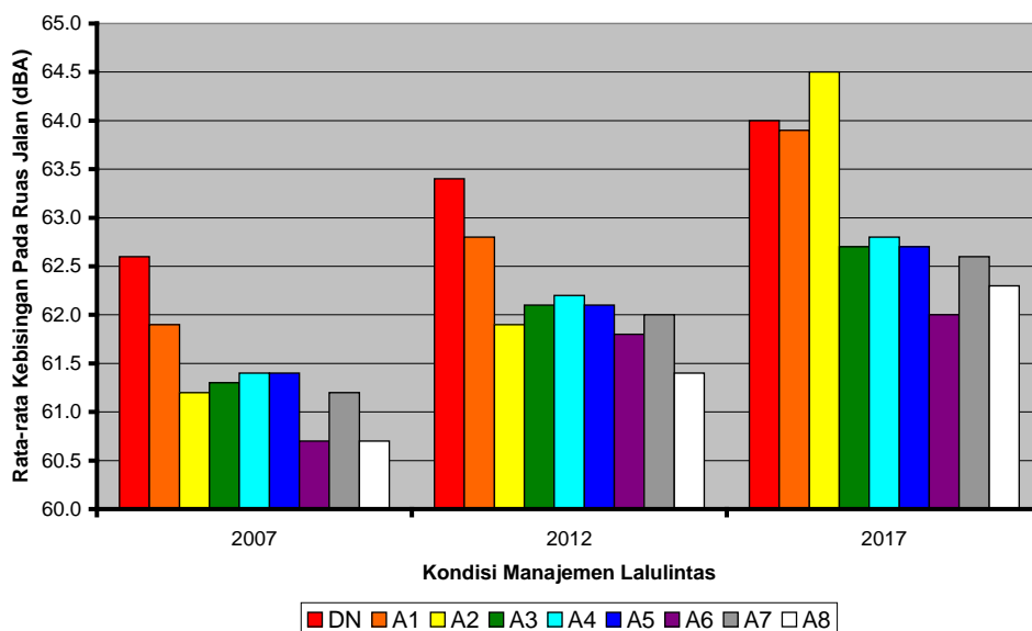
Gambar 14 Perbandingan Tingkat Kebisingan Rata-Rata Pada Ruas Jalan untuk Tahun 2007 Hingga Tahun 2017
