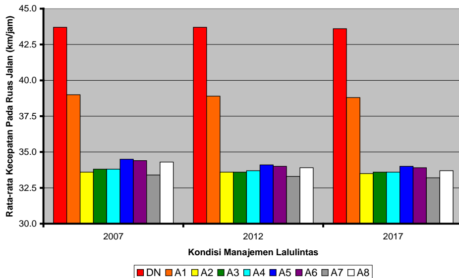
Gambar 10 Perbandingan Kecepatan Rata-Rata Pada Ruas Jalan untuk Tahun 2007 Hingga Tahun 2017
