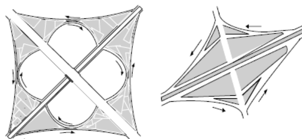
Gambar 5 Persimpangan Tak Sebidang
