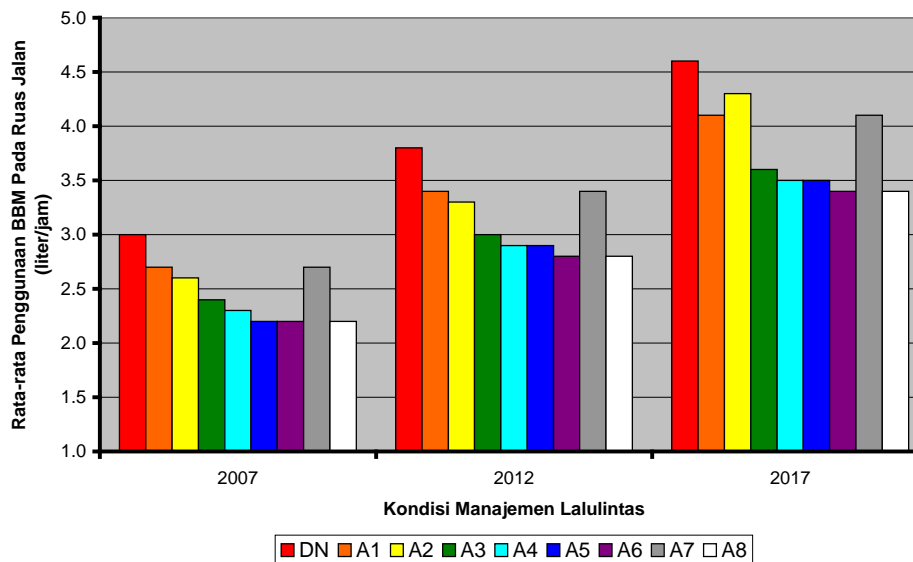
Gambar 12 Perbandingan Penggunaan BBM Rata-Rata Pada Ruas Jalan untuk Tahun 2007 Hingga Tahun 2017
