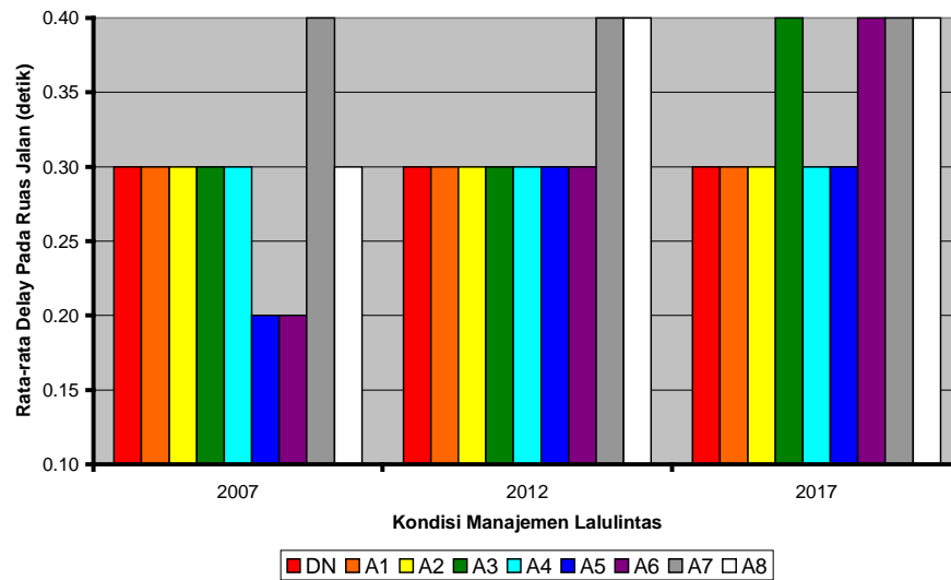
Gambar 9 Perbandingan Delay Rata-Rata pada Ruas Jalan untuk Tahun 2007 Hingga Tahun 2017
