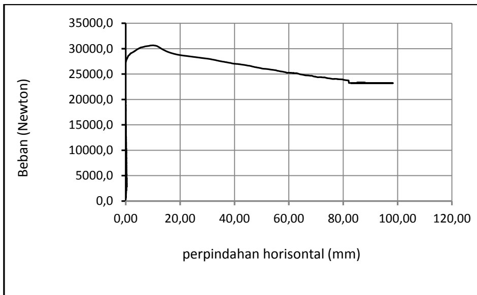
Gambar 4.14. Kurva Beban – perpindahan horisontal flens tertekan
