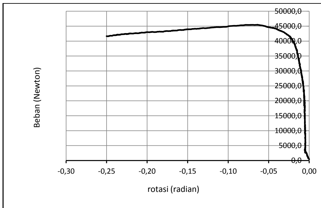
Gambar 4.30 Kurva beban-rotasi balok 2,8 meter berpegaku Dengan kemiringan 1:2
