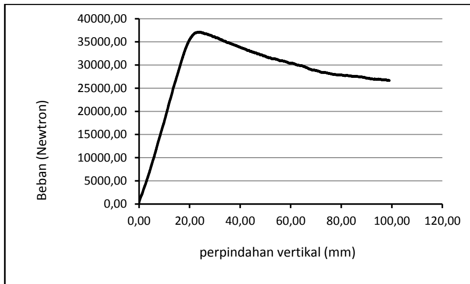
Gambar 4.22. Kurva beban-perpindahan vertikal balok 2,8 meter tanpa pengu
