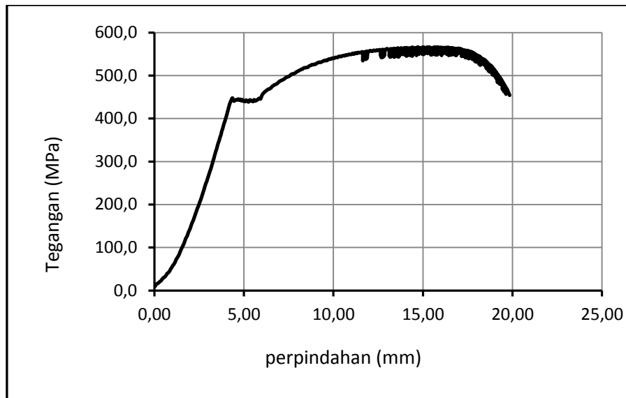
Gambar 4.12 Kurva tegangan – perpindahan B3
