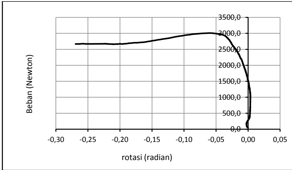
Gambar 4.21 Kurva beban-rotasi balok 3,8 meter berpengu
