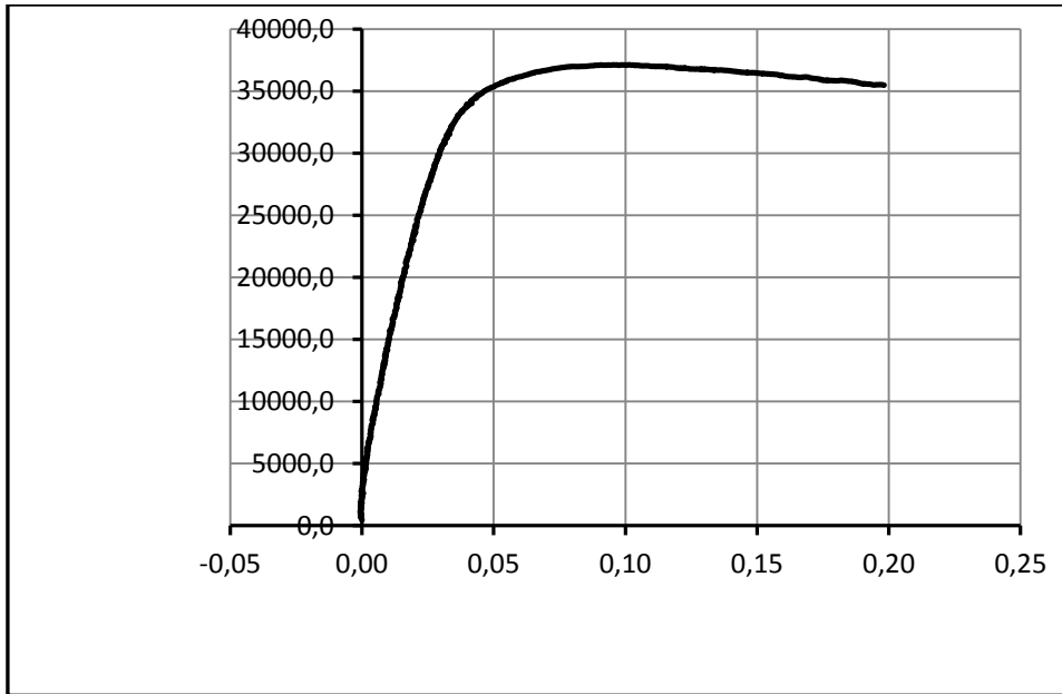
Gambar 4.23 Kurva beban perpindahan horisontal balok 2,8 meter tanpa pengaku
